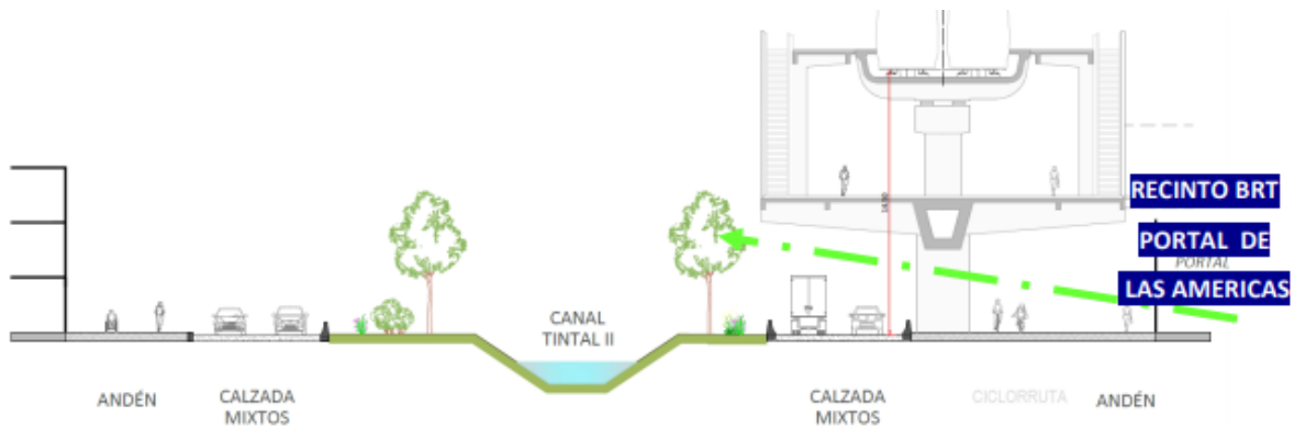
Figura 6.27 Sección tipo en el canal Tintal II con estación metro en conexión con Portal de las Américas – Fuente: SYSTRA
