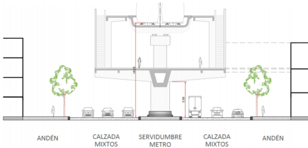
Figura 6.31 Sección tipo Av. Villavicencio con estación Villablanca – Fuente: SYSTRA
