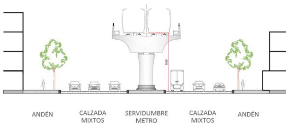
Figura 6.34 Sección tipo Av. Primero de Mayo con inserción central sobre separador existente – Fuente: SYSTRA
