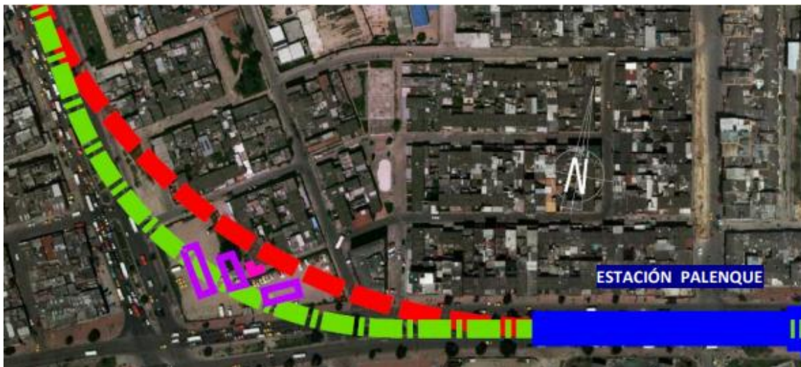
Figura 6.32 Planta con enlace entre Av. Villavicencio y Av. Primero de Mayo: trazado aéreo R200 en verde y subterráneo R325 en rojo, estación de servicio existente en violeta – Fuente: SYSTRA
