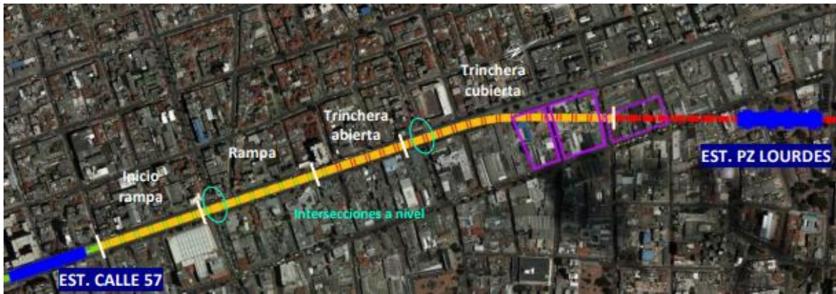
Figura 6.20 Transición infraestructura elevada a subterránea Alternativa Familia C – Fuente: SYSTRA
