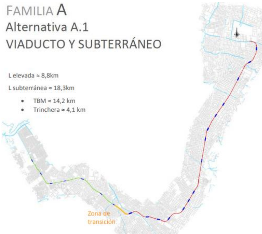
Figura 6.11 Alternativa A.1 – Fuente: SYSTRA
