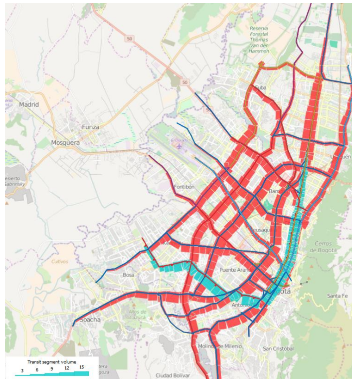
Figura 6.88 Diagrama de carga en la red de transporte masivo simulada en la HP 2030 – Fuente: SDM
