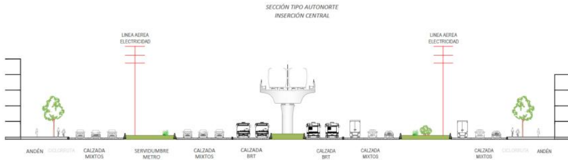
Figura 6.57 Sección tipo Autonorte con inserción central sobre el separador de Transmilenio – Fuente: SYSTRA
